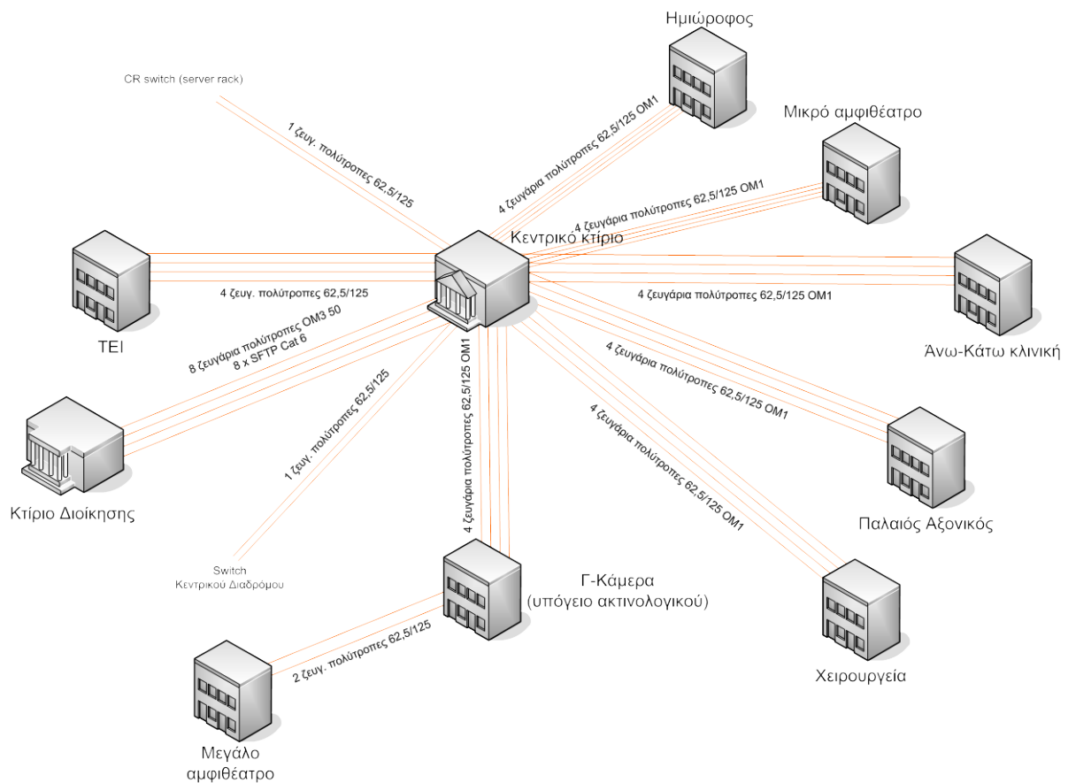
Σχήμα 2: Εγκατεστημένες οπτικές ίνες.
