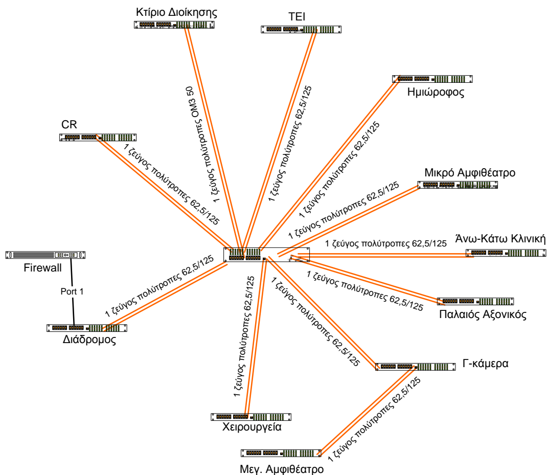
Σχήμα 1: Τοπολογία LAN
